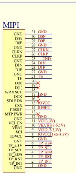
MIPI接口参考接线图
