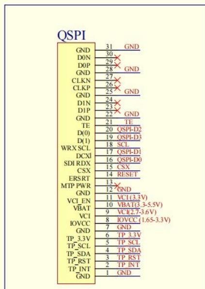
QSPI接口参考接线图
